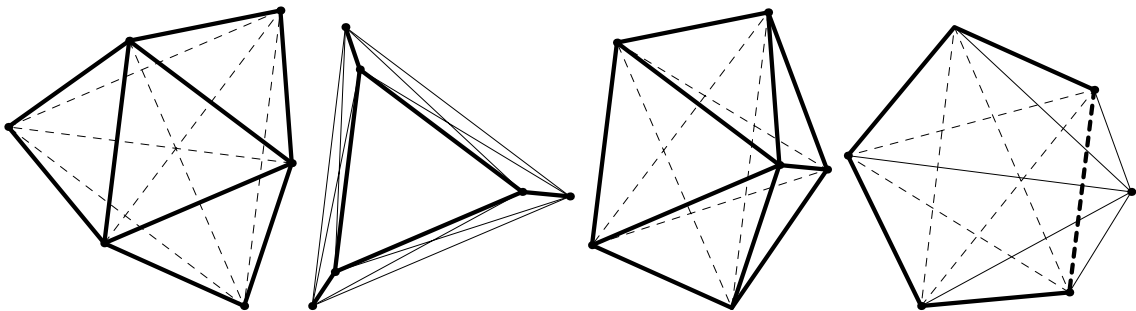
Рис. 4 Четыре примера множеств с двумя расстояниями получающимися из правильного икосаэдра. Жирные линии обозначает расстояния равные 1, а тонкие \sqrt{5}/2 .
