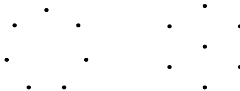
Рис. 5 Множества из 7-ми точек на плоскости, между которыми только три вида расстояний.
